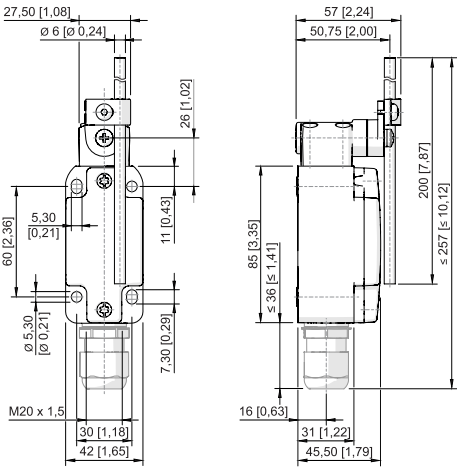
Rod lever 8070/2-DD-U60
