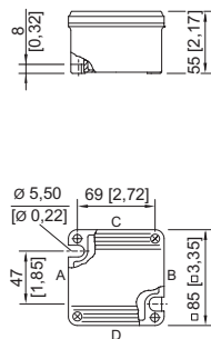
8118/.1. Enclosure SZ 1
