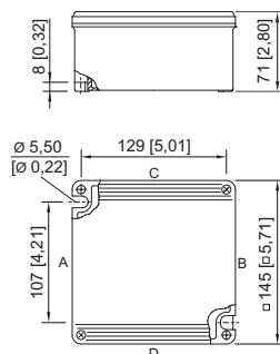
8118/.3. Enclosure SZ 3
