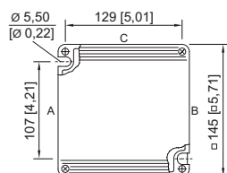
8118/3. Enclosure SZ 3
