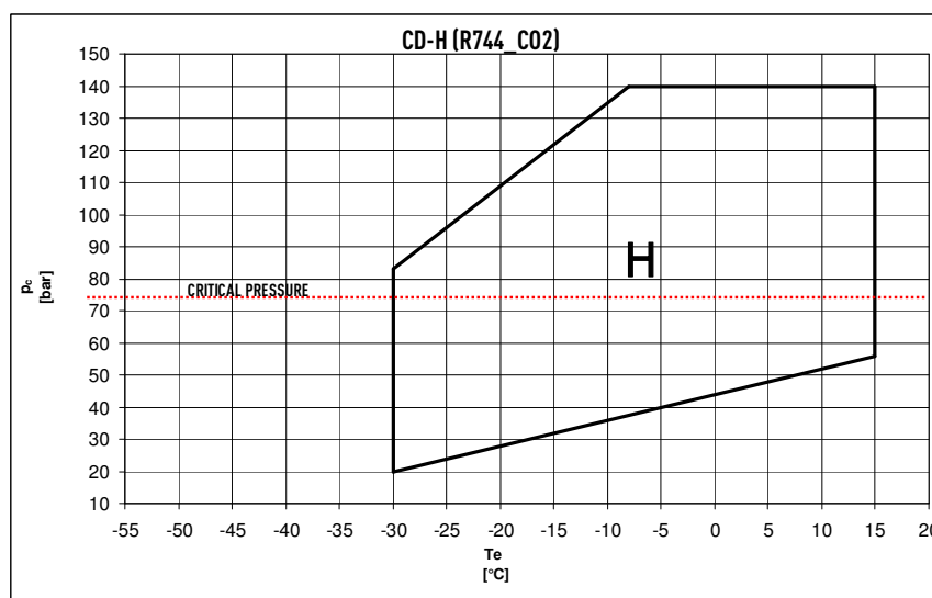
Fig. 4: CD200, CD300, CD400 - Limiti d'applicazione – Application limits – Champs d'application
