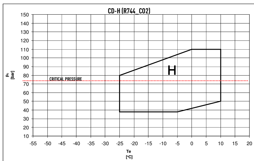
Fig. 4: CD500 - Limiti d'applicazione – Application limits – Champs d'application
