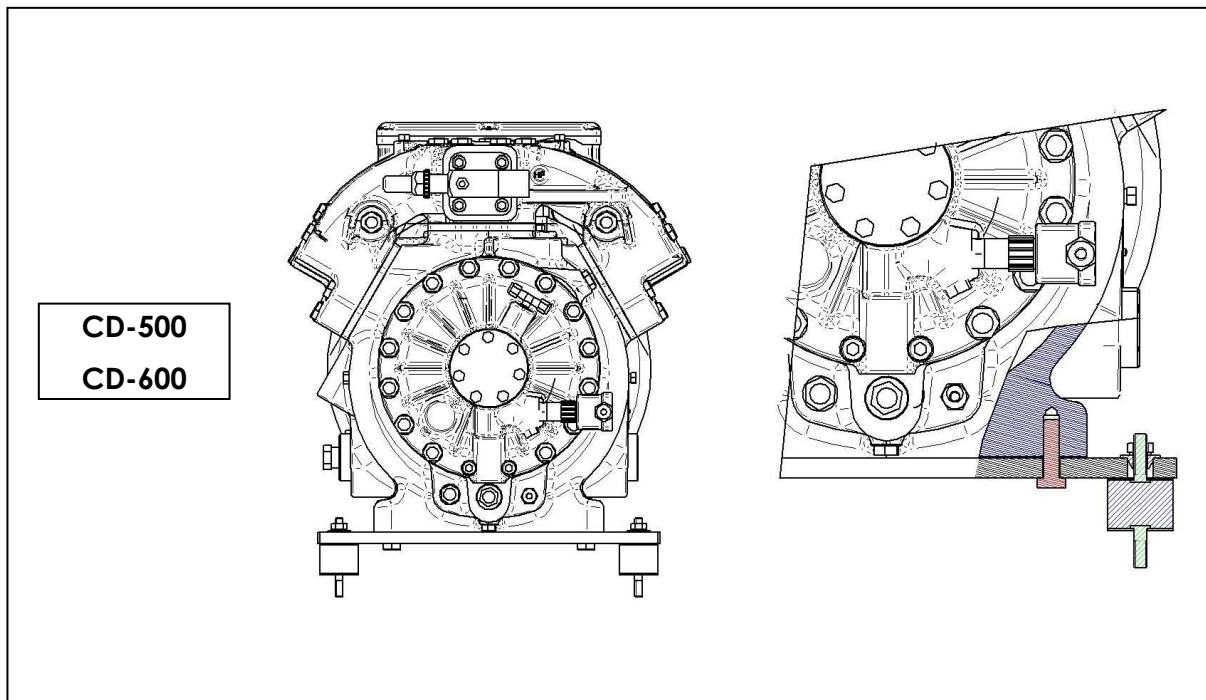
Fig. 2: Impiego degli antivibranti - Vibrational dampers use - Utilisation du support amortisseurs
