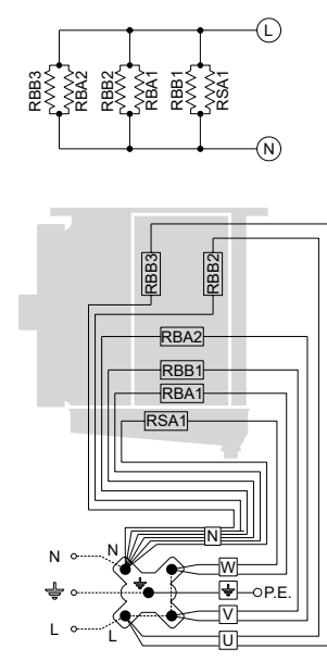
Connexion 230V/1/50-60Hz à predisposer
