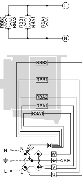
Connexion 230V/1/50-60Hz à prédisposer
