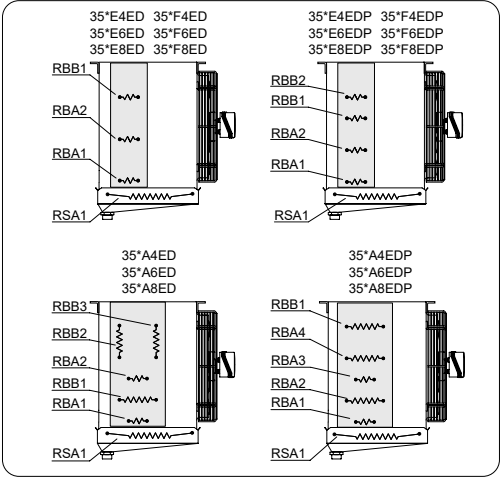
Détail de positionnement résistances
