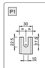
Détail de fixage
