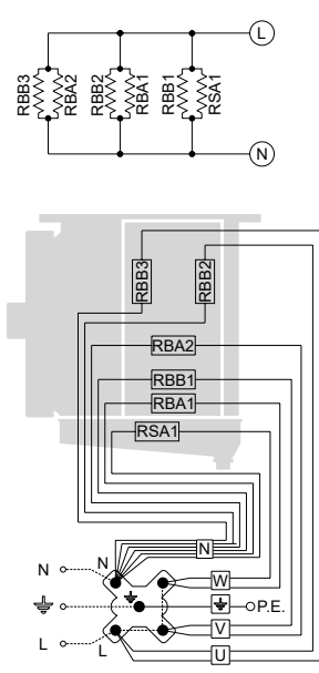
Collegamento 230V/1/50-60Hz da predisporre
