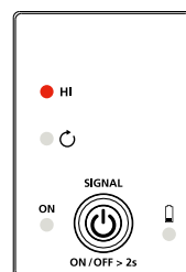
Figura 3.1c: Indicador del transmisor que muestra la señal en el modo HIGH (ALTO)
