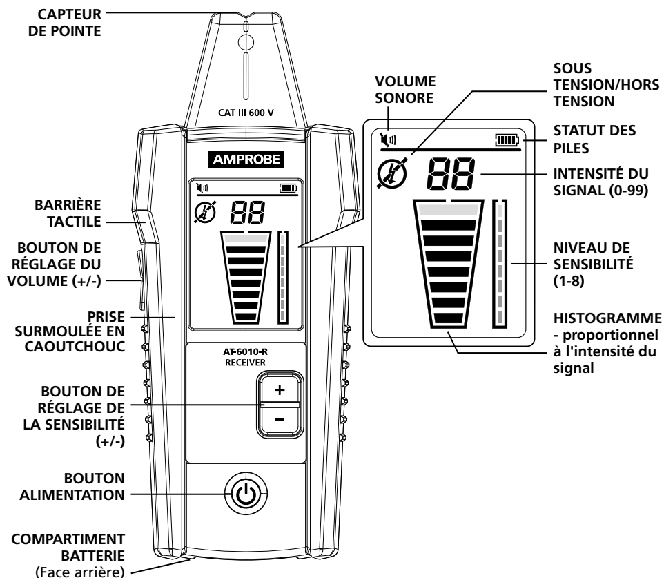
Figure 2.1 : Vue d'ensemble du récepteur AT-6010-R
