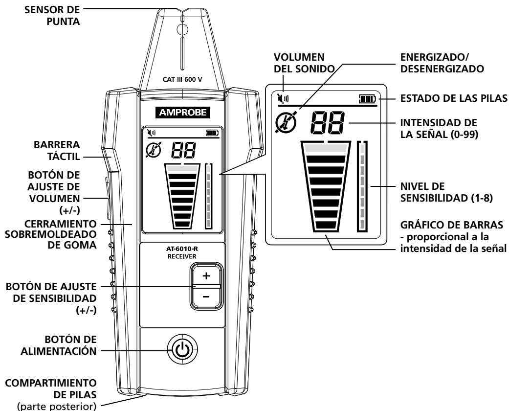
Figura 2.1: Descripción general del receptor AT-6010-R
