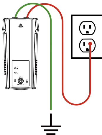
Figura 3.2b: Conexión a tierra independiente (preferida)
