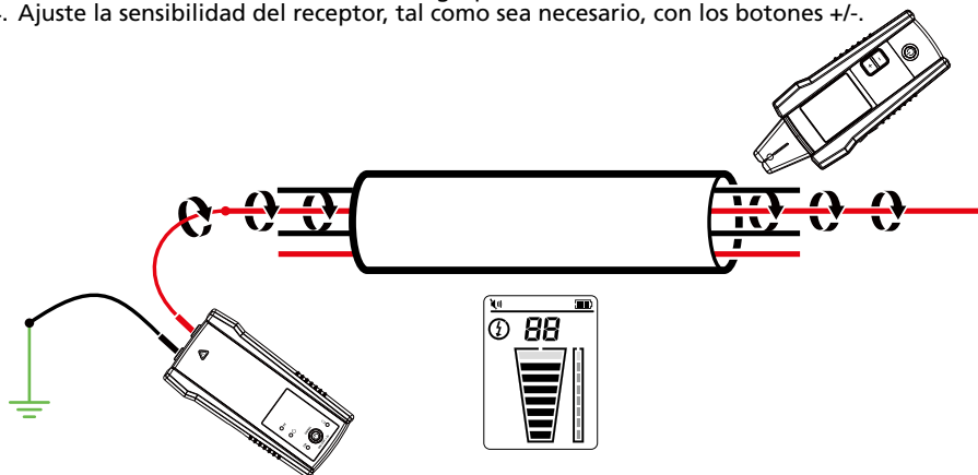
Figura 4.9: Identificación de un cable específico en un grupo
