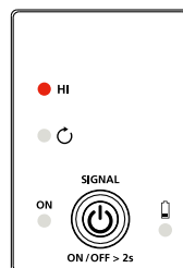
Figure 3.1c : Indicateur du transmetteur affichant le signal en mode ÉLEVÉ
