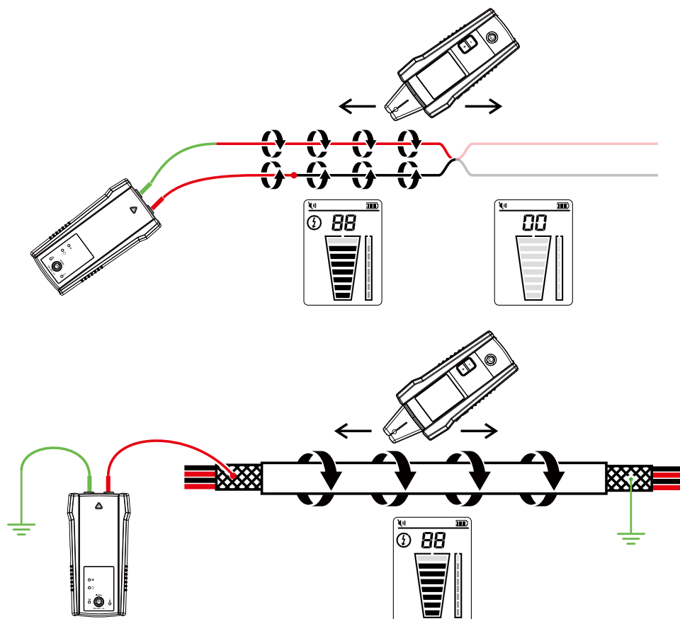
Figure 2.2b : Générer un signal en mode Boucle
