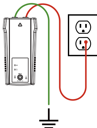
Figura 3.1a: Conexión adecuada con conexión a tierra independiente
