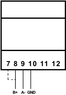
Modbus RTU: RS485 Slave (last device)
