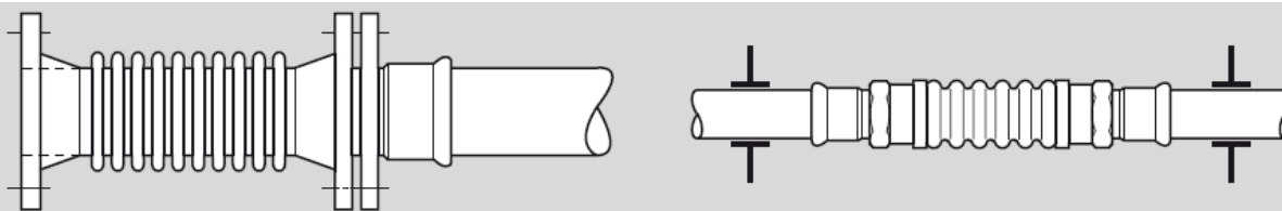
Fig. 12 Compensatori di dilatazione assiali axial expansion compensators
