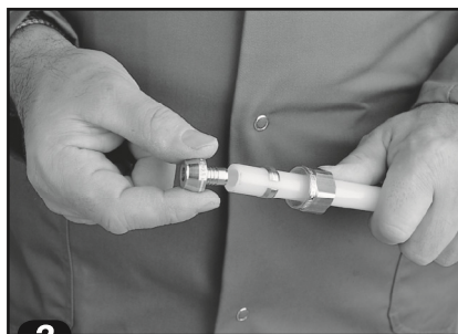
2 Monter omløber, klemring og støttebøs- ning på Pex-røret i nævnte rækkefølge. Koblingen sammenspændes i.h.t koblings- fabrikantens anvisning.
