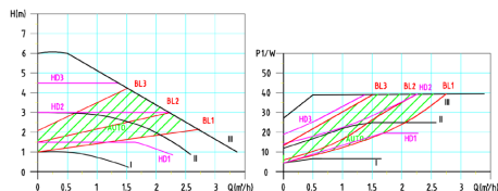
EPxx-60-xx ydelseskurve
