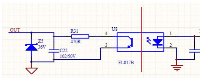
PWM-udgangsinterfacekredsløb
