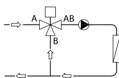
Fig. 2: Blandeventil anvendt i blandefunktion
