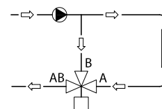
Fig. 3: Blandeventil anvendt i fordelerfunktion
