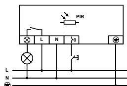
Tilslutningsskema
