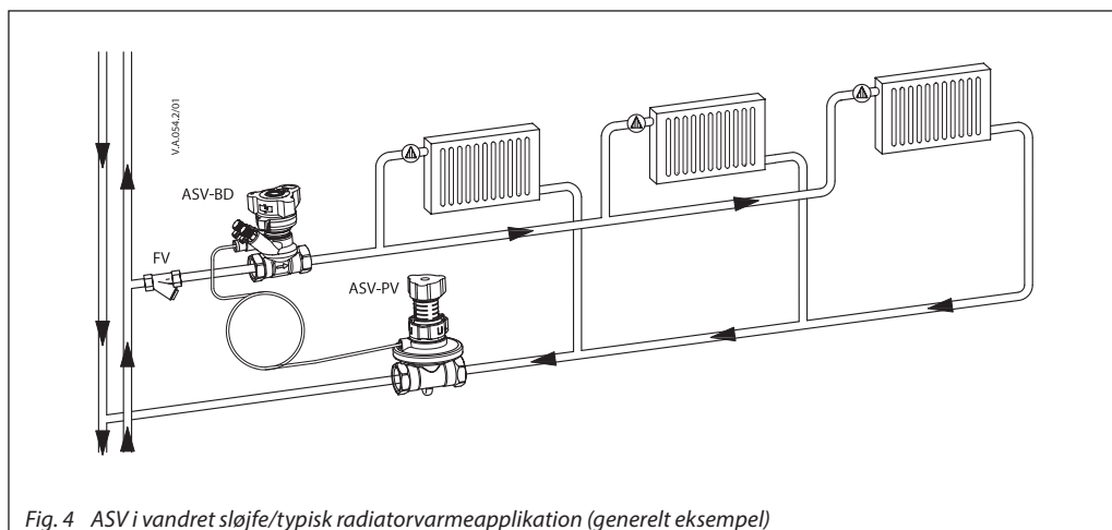
Fig. 4 ASV i vandret sløjfe/typisk radiatorvarmeapplikation (generelt eksempel)
