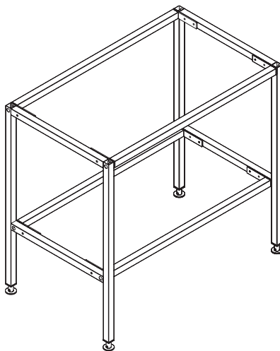
Eksempel: stativ til 1000 mm bordplade
