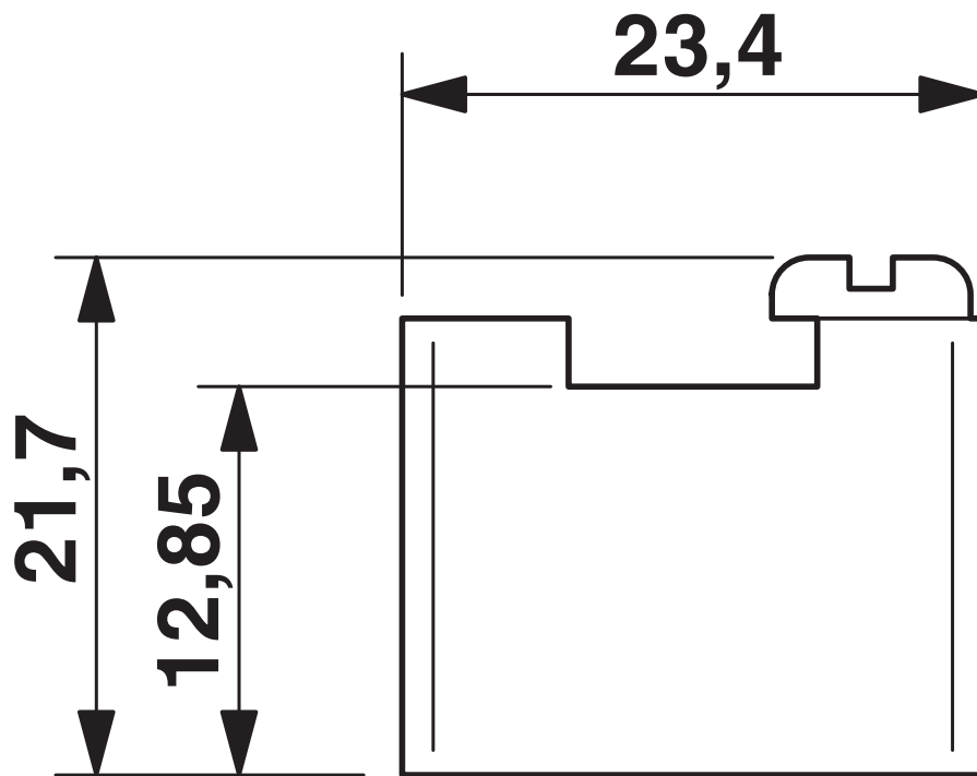
Målskitse
