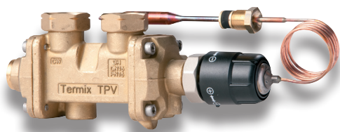
Termix TPV 90 anvendes i vandvarmeren Termix Novi
