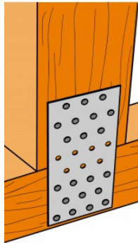
T-samling ved hjælp af NP hulplade
