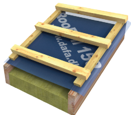
Ventileret undertag
