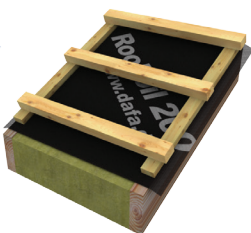
Diffusionsåbent undertag
