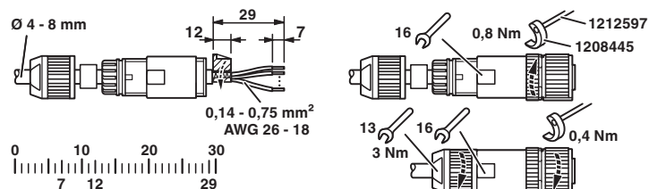
Funktionsskitse
