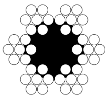
Galv. Stålwire, konstruktion 6x7+1FC Galv. Steel Wire Rope, Construction 6x7+1FC
