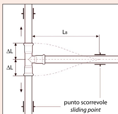
Fig. 16 Derivazione a T T-shaped branch
