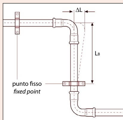
Fig. 15 Compensatori di dilatazione a Z Z-shaped expansion compensators
