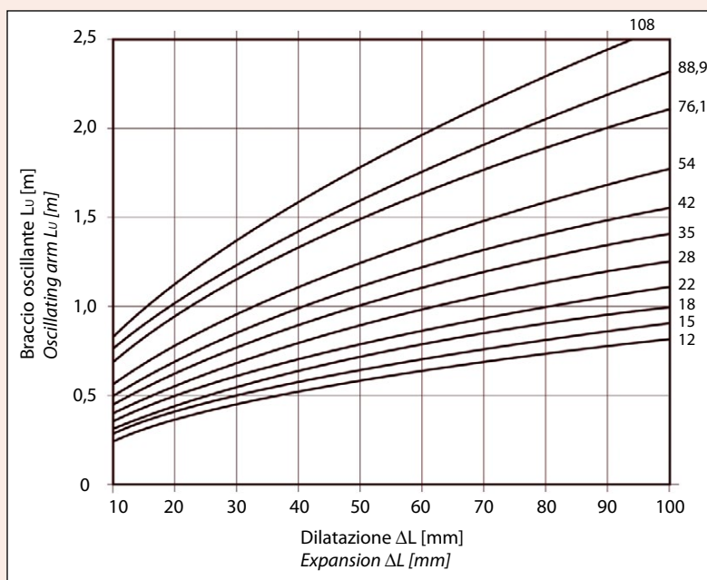
Fig. 14 Lunghezza L_u del compensatore ad U in acciaio inossidabile Length L_u of U-shaped compensator in stainless steel
