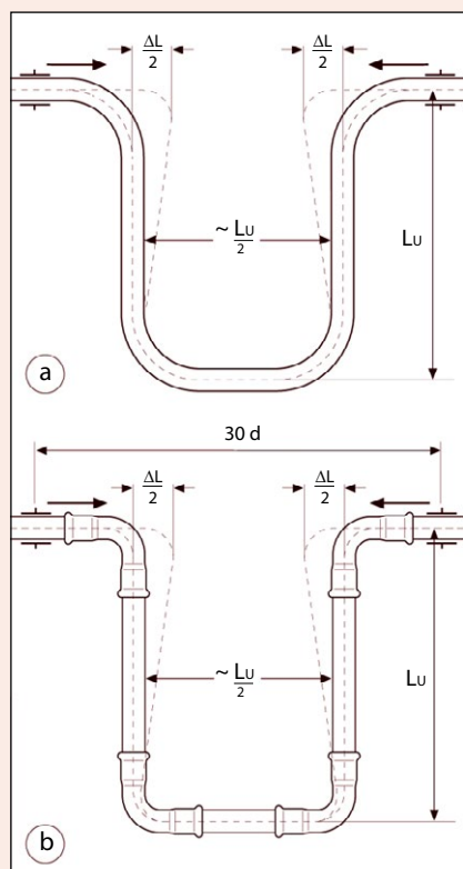
Fig. 13 Compensatori di dilatazione ad "U" U-shaped expansion compensators a) in tubo preformato a) through preformed pipe b) con raccordi pressfitting b) with pressfittings
