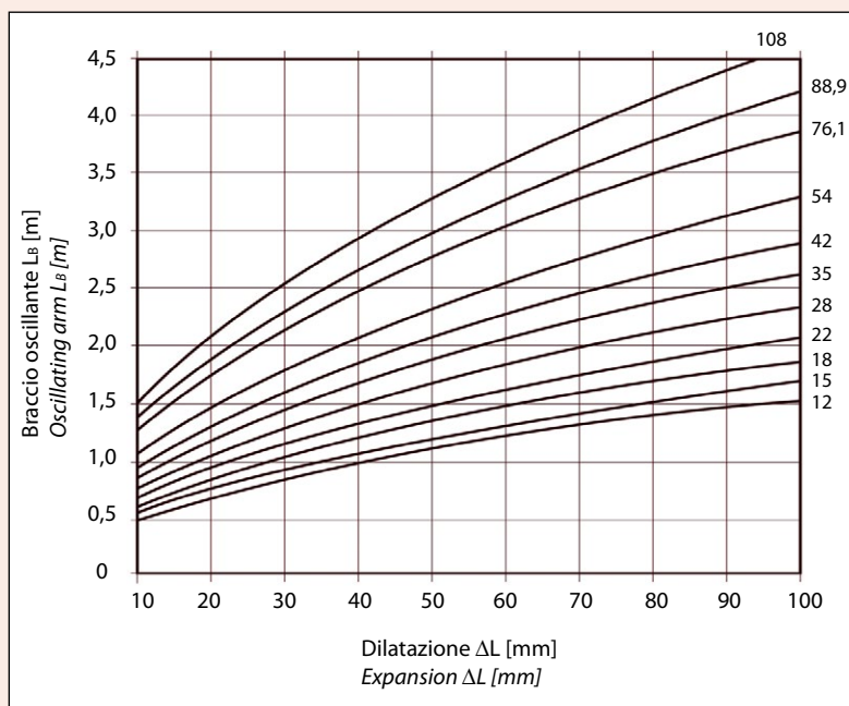
Fig. 17 Lunghezza L_B del compensatore a Z in acciaio inossidabile Length L_B of Z-shaped compensator in stainless steel
