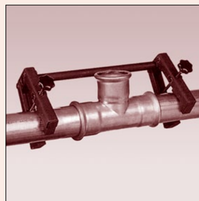
Fig. 26 Utilizzo della morsa di montaggio per diametri "Big Size". Use of assembly clamps for "Big Sizes" diameters
