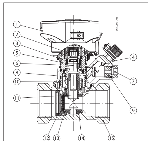
Fig. 7 ASV-BD DN 15-50
